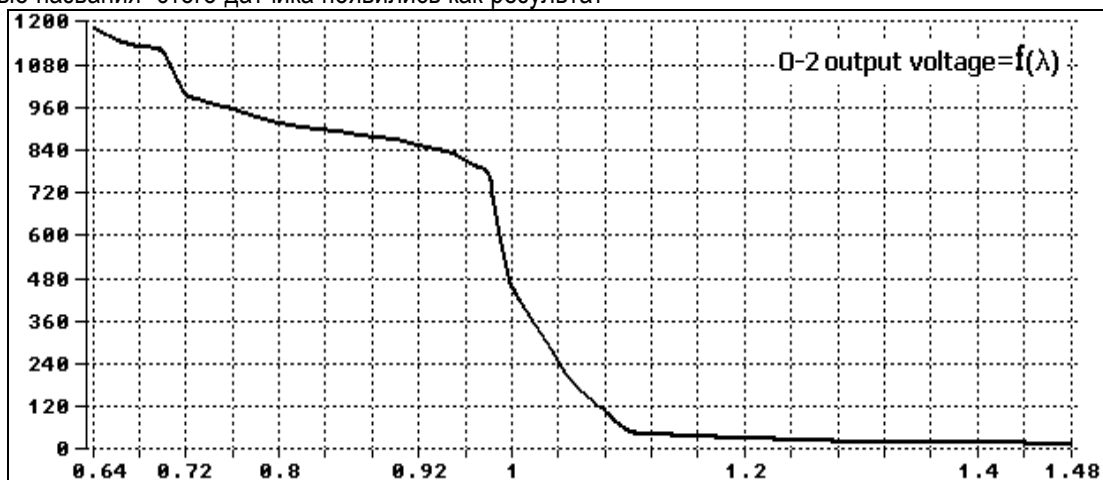
Выходная характеристика циркониевого Лямбда-зонда.
